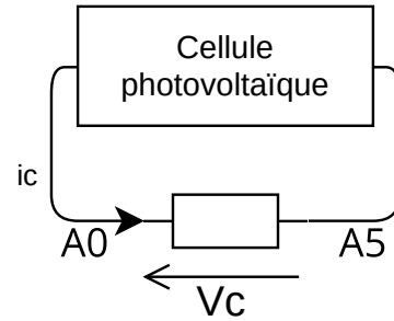
(c) Schéma théorique de la cellule photovoltaïque
